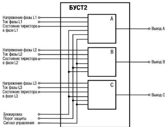
Рисунок 6.4 – Каналы управления тиристорами
